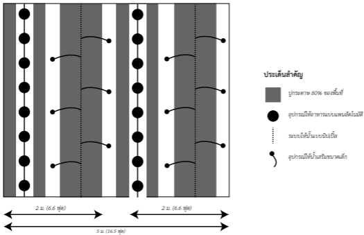
รูปแบบทั่วไปแบบระบบกกลูกไก่ทั้งโรงเรือน (ต่อลูกไก่ 1,000 ตัว)
