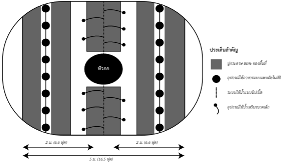
รูปแบบจุดกกแบบหัวกกทั่วไป (ต่อลูกไก่ 1,000 ตัว)
